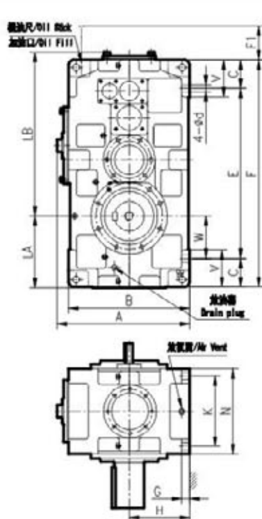
P系列TSG齒輪箱外形尺寸圖 TSG Gear Box Size Chart for Parallel Shaft
