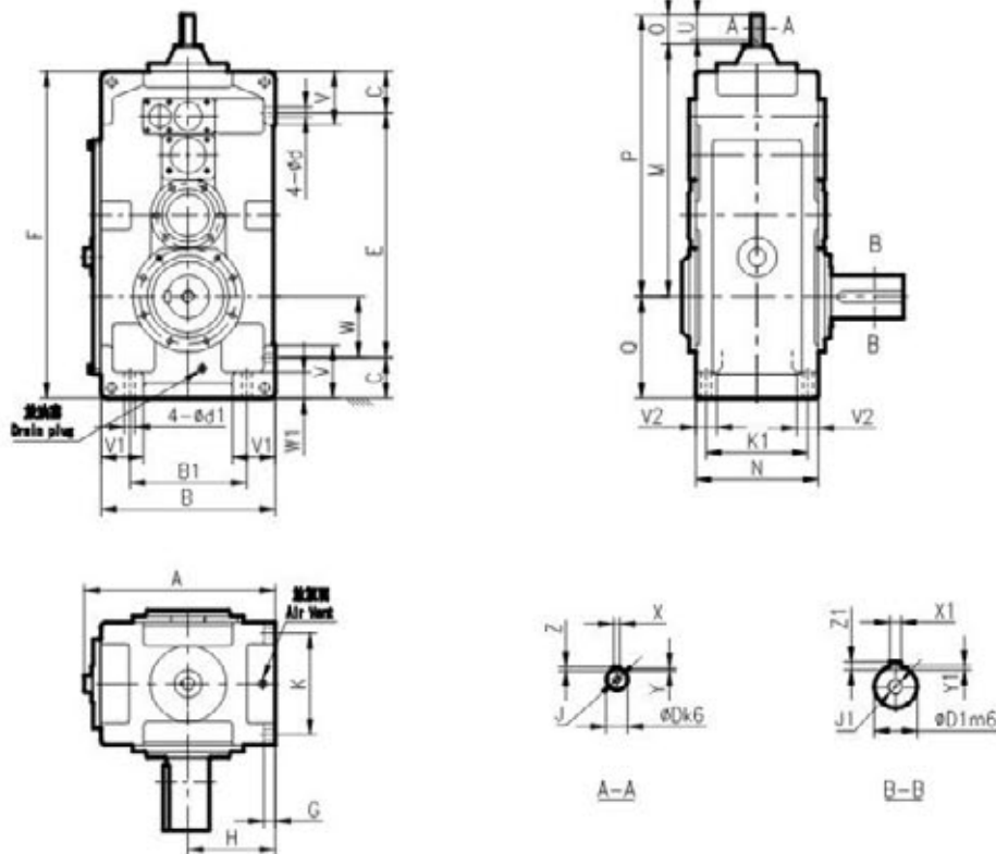
R系列TSG齒輪箱外形尺寸圖 TSG Gear Box Size Chart for Right Angle Shaft
