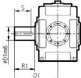
實心出力軸 Solid Output Shaft
