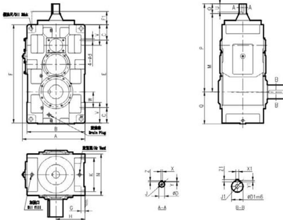
R系列TSG齒輪箱外形尺寸圖 TSG Gear Box Size Chart for Right Angle Shaft
