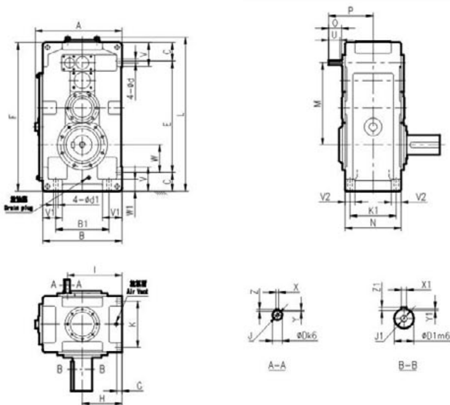
P系列TSG齒輪箱外形尺寸圖 TSG Gear Box Size Chart for Parallel Shaft
