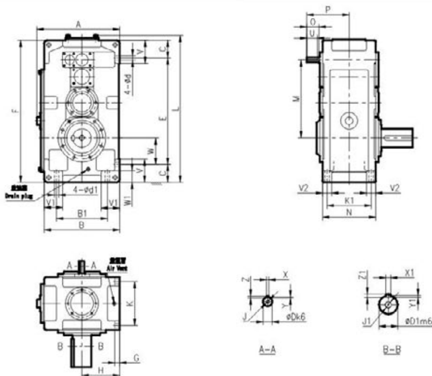
P系列TSG齒輪箱外形尺寸圖 TSG Gear Box Size Chart for Parallel Shaft
